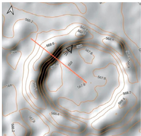
▲ Lidarové zachycení starého milíře v lesním porostu a jeho reálné odkrytí v terénu s patrnými pozůstatky dřevěného uhlí. Foto L. Šefrna
